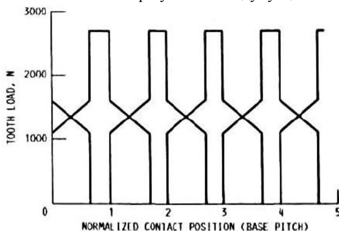
Рис. 1. Цикли навантаження зубців зубчастого колеса
