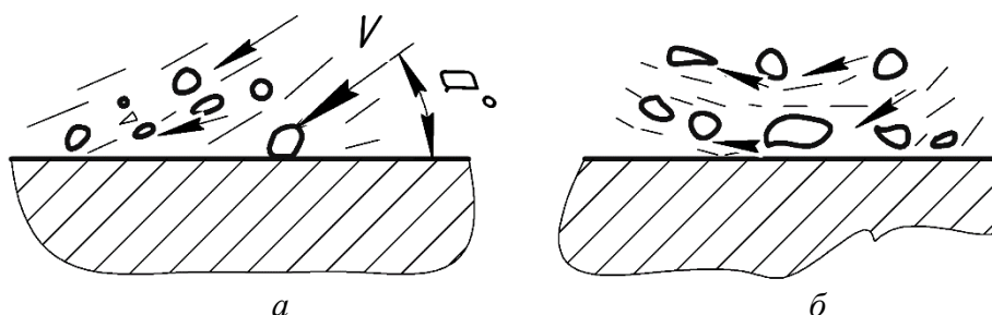
Рис. 2. Схеми зношування:
