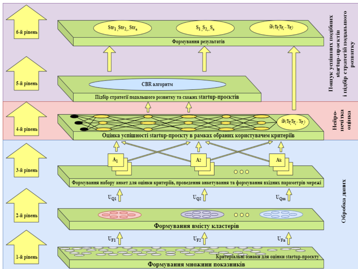
Рис. 1. Концептуальна схема нейро-нечіткої моделі інформаційної технології комплексної оцінки рівня успішності startup-проєктів
