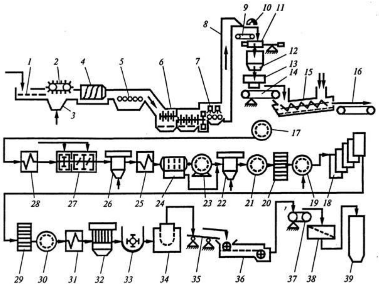
Машино-апаратурна схема лінії виробництва хлібопекарських дріжджів
