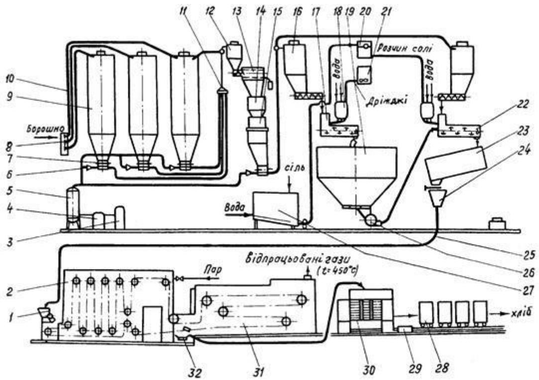
Машинно-апаратурна схема виробництва хліба формового
