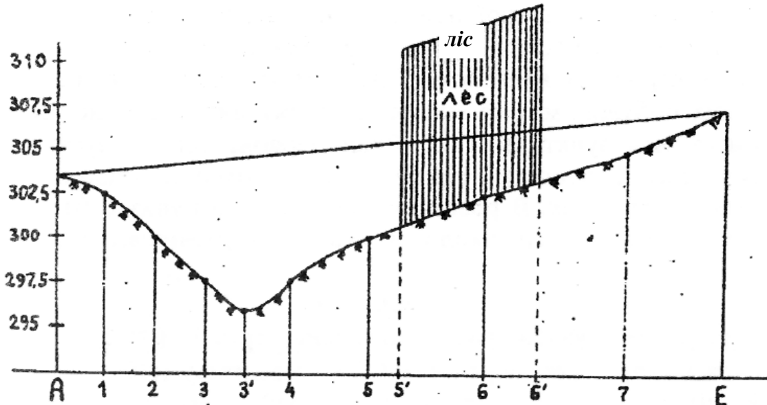
Рис. І.2.3. Профіль між точками A і E
