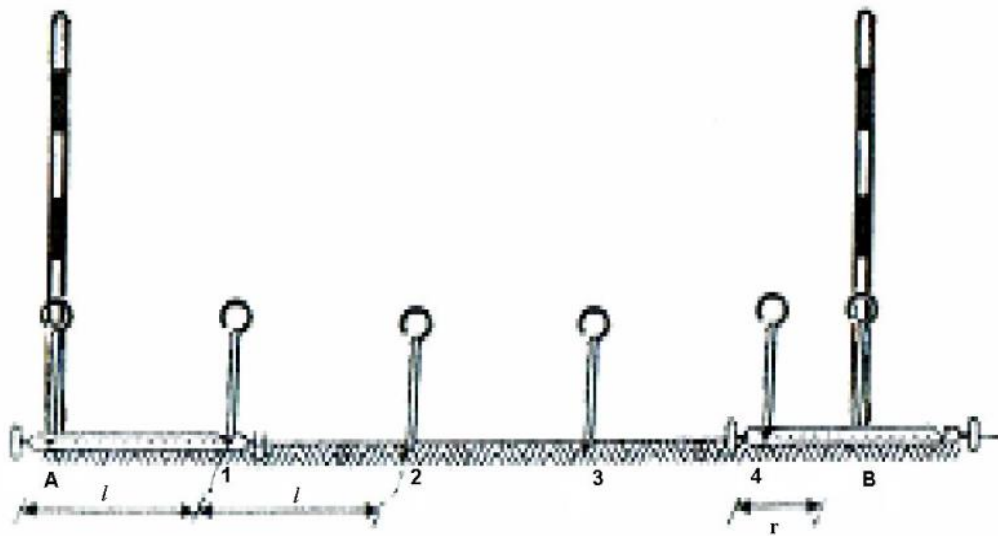
Рис.І.4.4. Вимірювання ліній стрічкою
