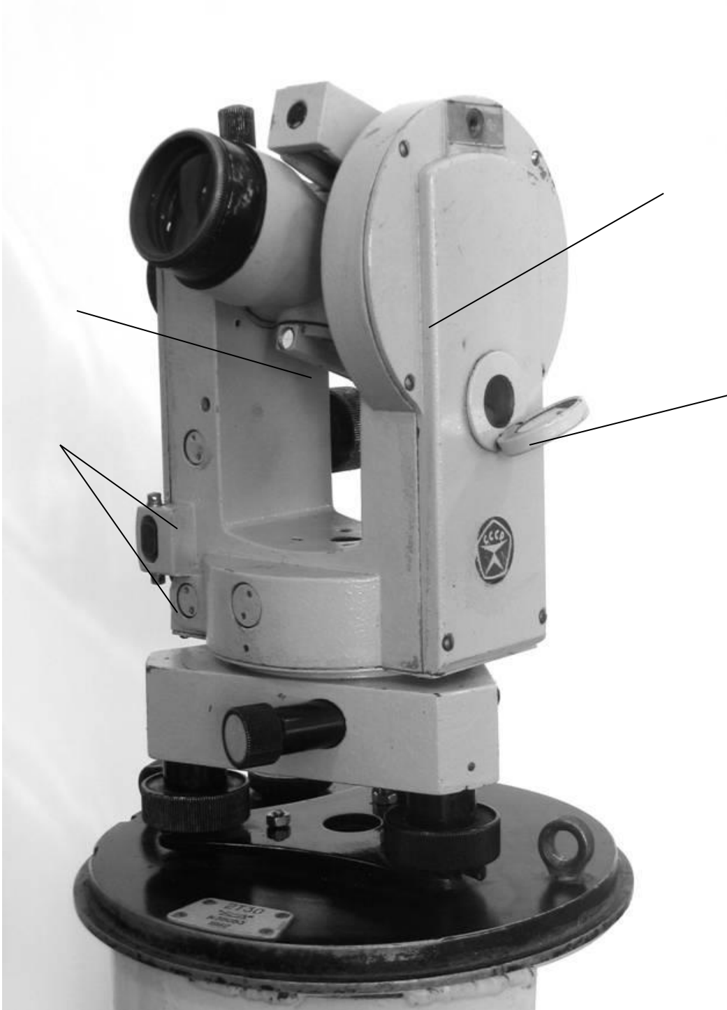
Рис. II.1.1. Теодоліт 2Т30 (з боку вертикального круга)
