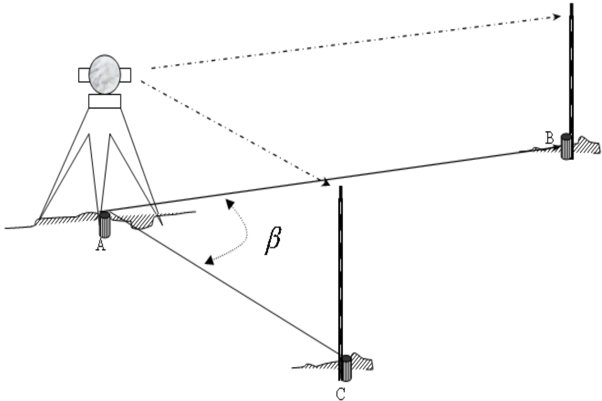
Рис. П.2.1.Схема вимірювання горизонтального кута
