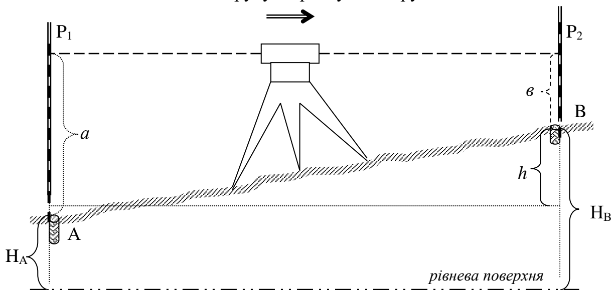
Рис. III.2.1. Геометричне нівелювання зі середини
