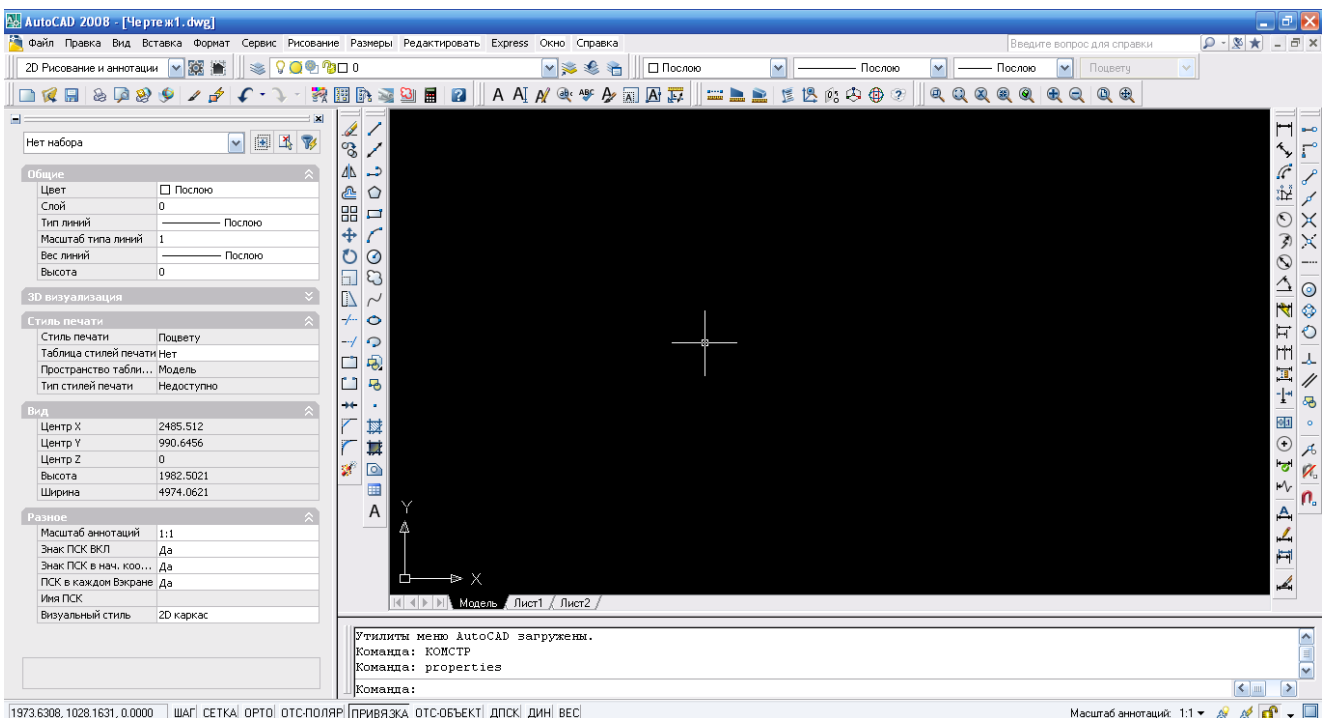
Рис. IV.4.1. Интерфейс AUTOCAD
