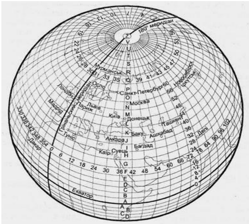
Рис. І.3.1. Схема розграфлення аркушів карти масштабу 1:1 000000
