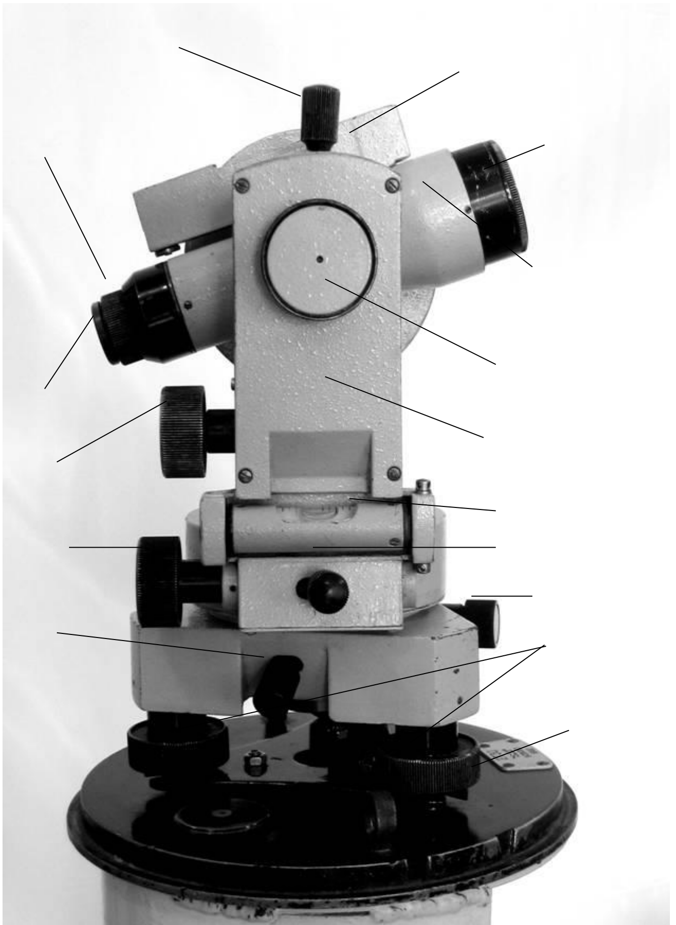
Рис. П.1.2. Теодоліт 2Т30 (з боку колонки)
