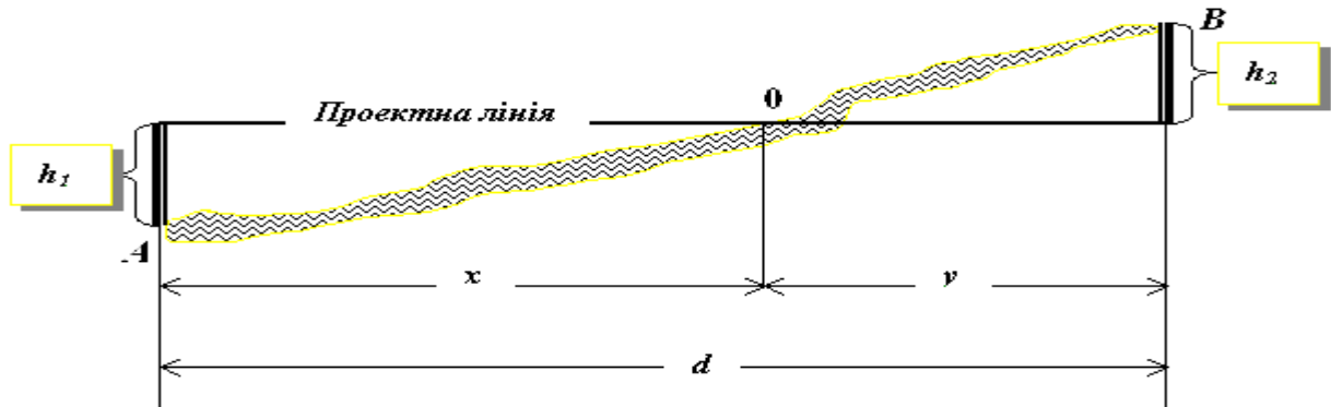
Рис. III.3.1. Точки нульових робіт на профілі
