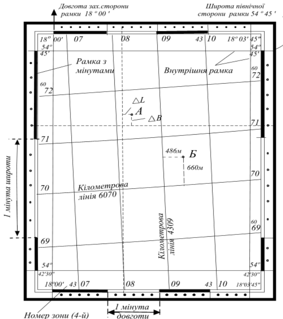
Рис. І.1.5. Визначення прямокутних та геодезичних координат
