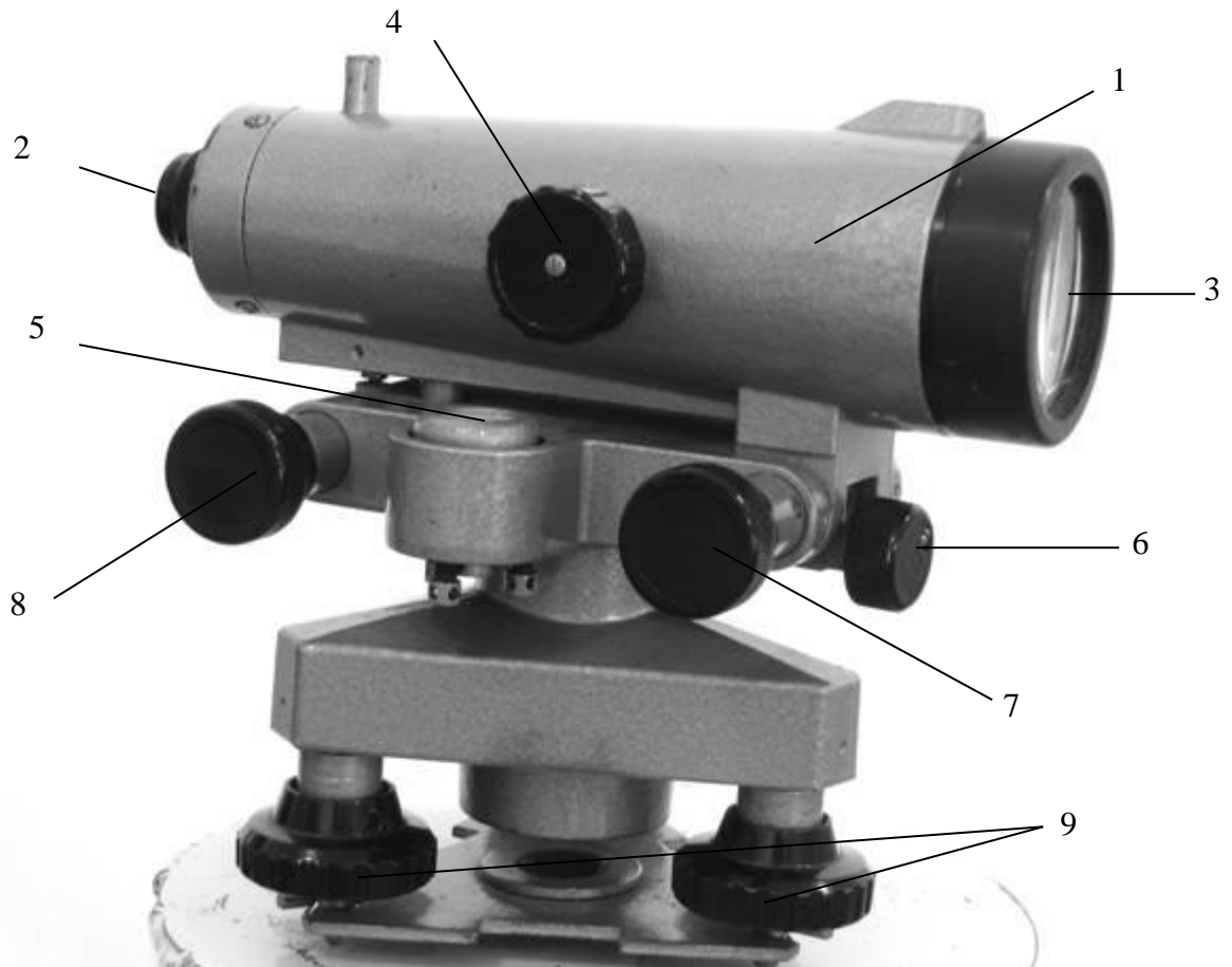
Рис. III.1.2 Нівелір Н-3 (а)
