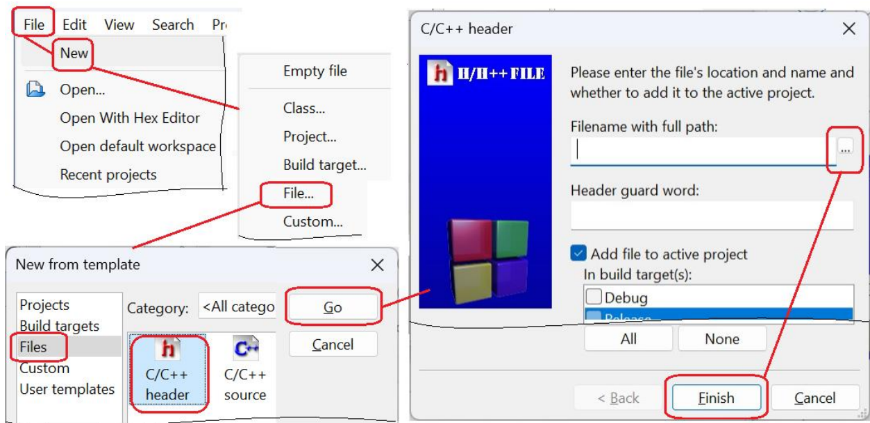
Рисунок 4 – Послідовність діалогових вікон для створення type.h
