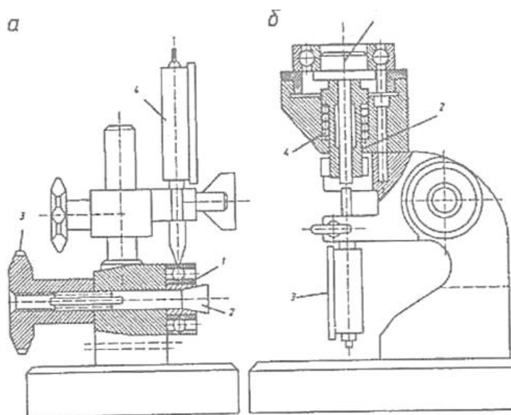
Рис. 1. Пристрої для контролю: а – радіального зазору в кульковому підшипнику; б – осьового зазору в кульковому підшипнику
