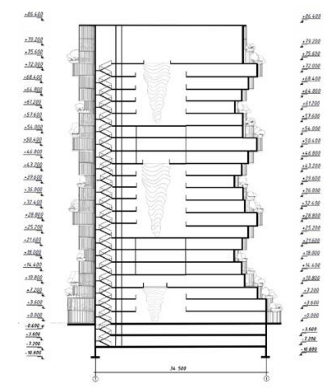
Розріз 1-1
