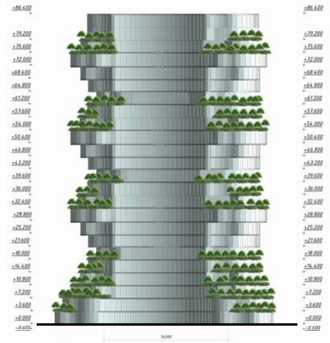
Фасад А-Ж
