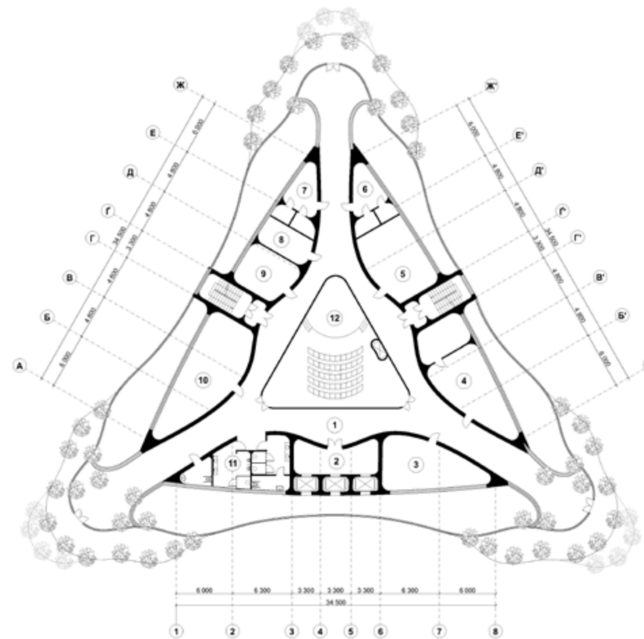
План творчої зони
