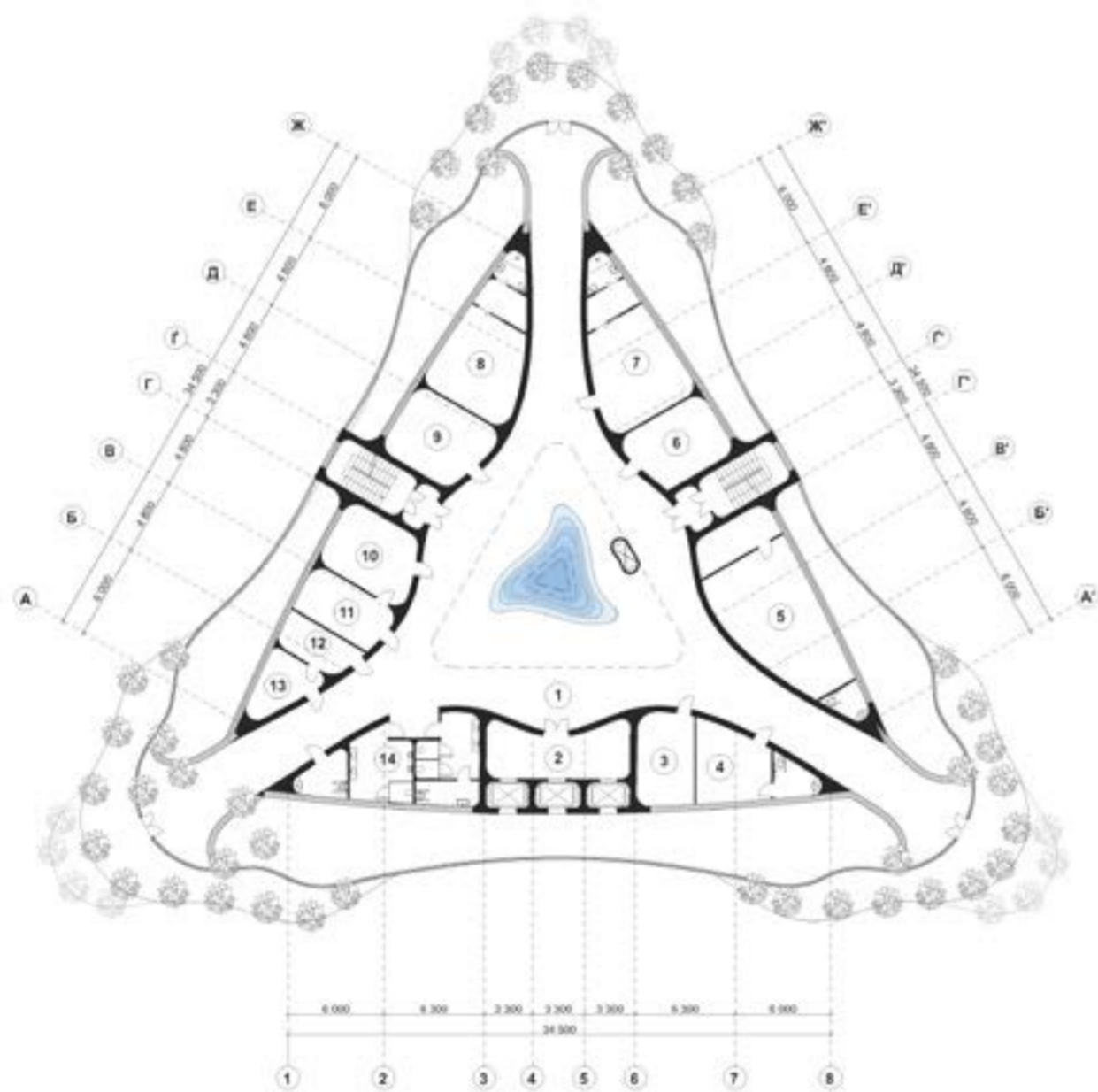
План оздоровчої зони
