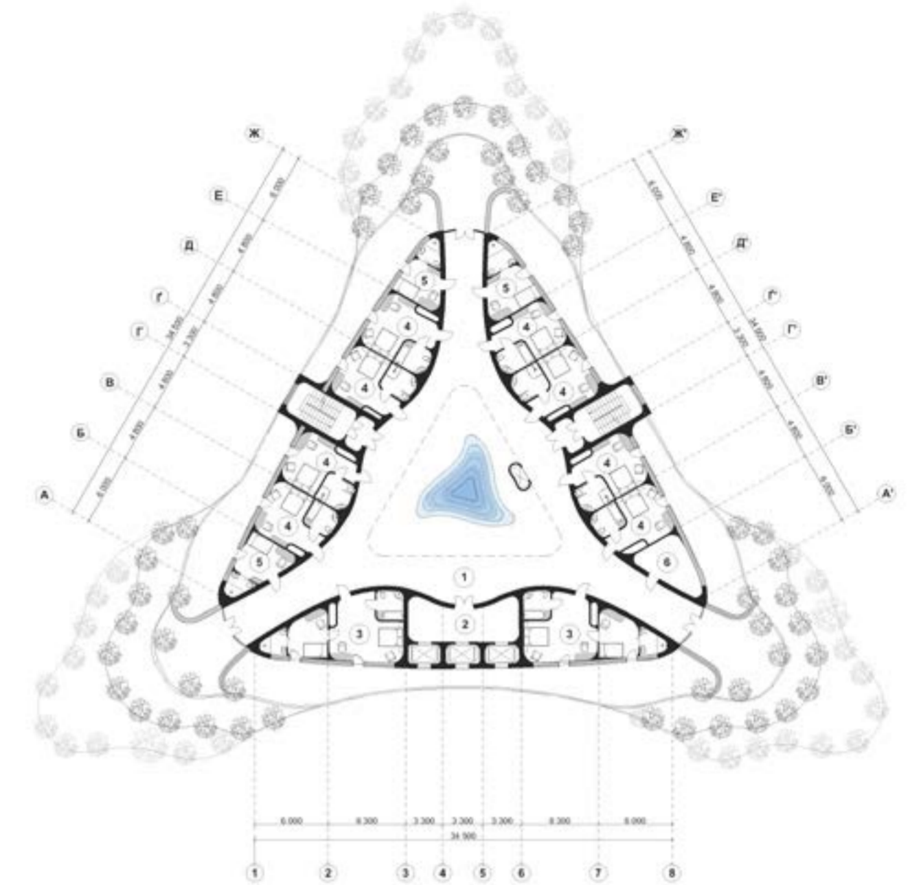
План житлової зони
