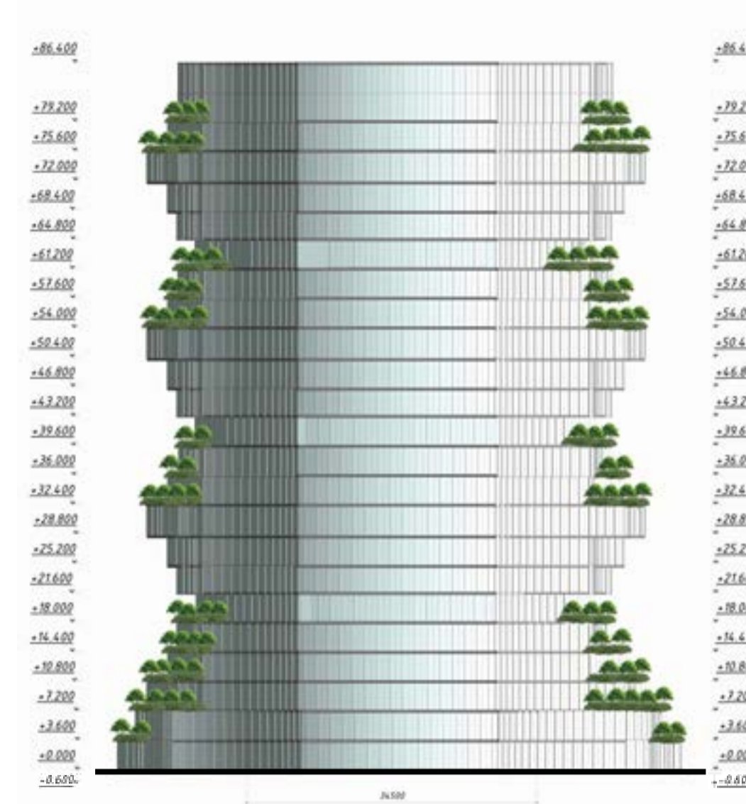
Фасад 8-1
