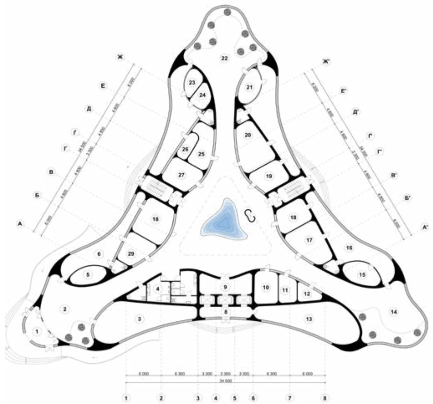
План 1-го поверху
