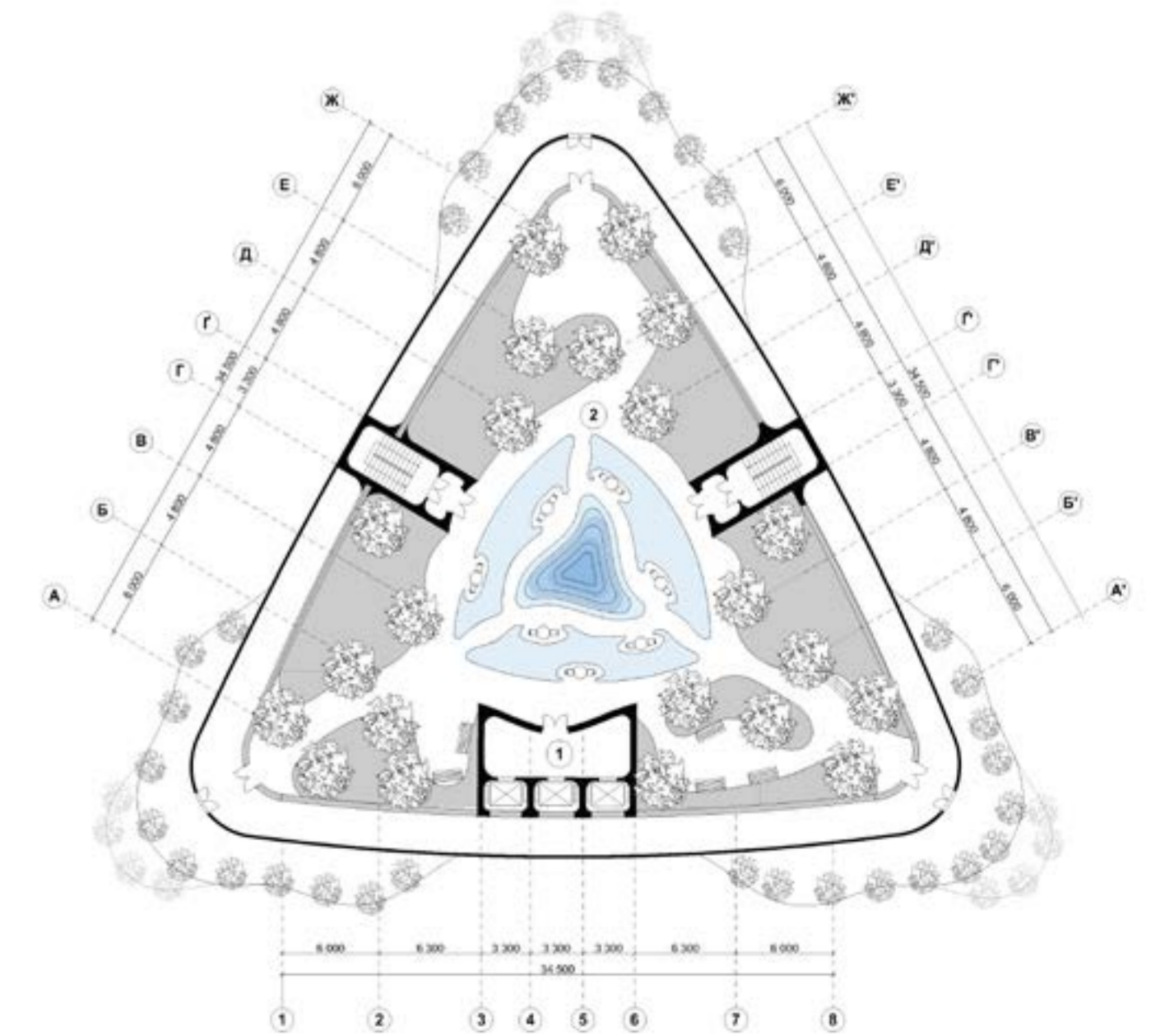
План зимового саду
