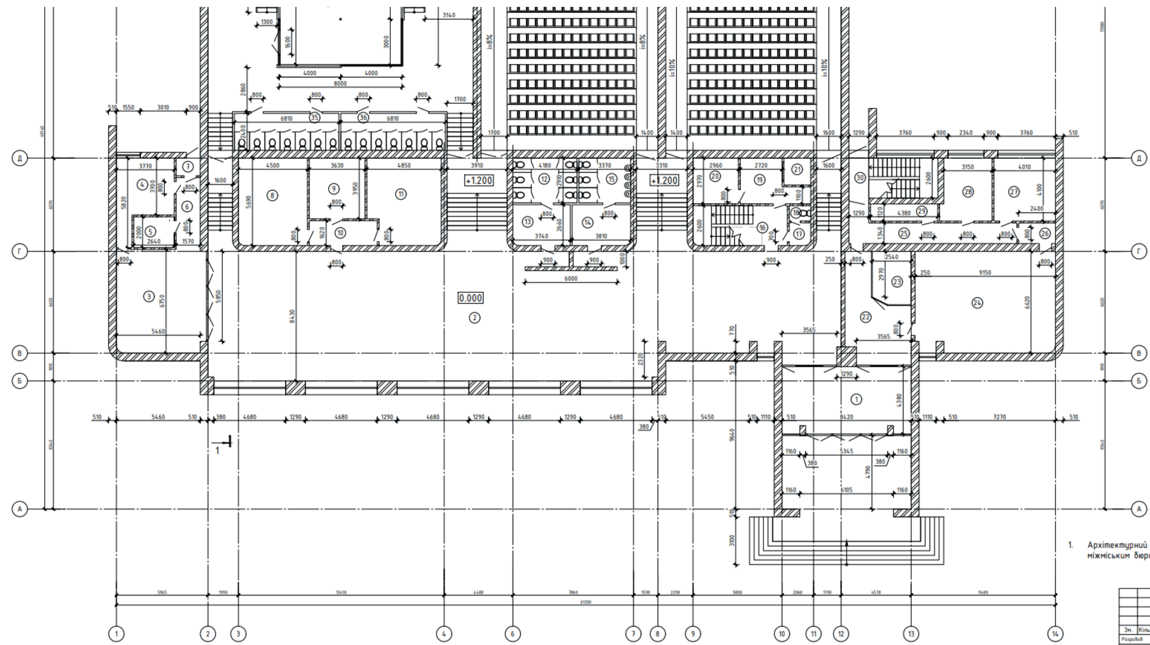
Архітектурний план
