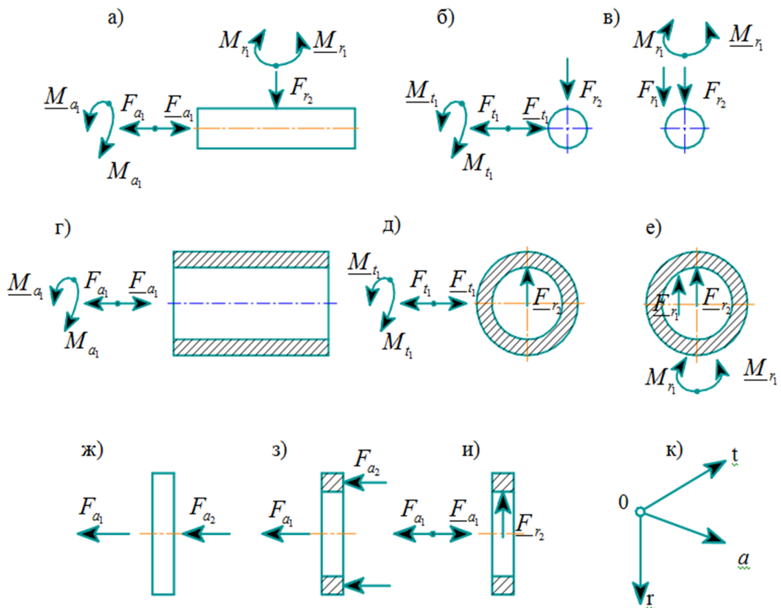
Рис. 3. Варіанти можливих силових потоків у захватних пристроях для маніпулювання суцільними циліндричними (а-в) та пустотілими циліндричними (з-е) деталями, суцільними дисками (ж) та кільцями (з-и) у циліндричній системі координат art (к)
