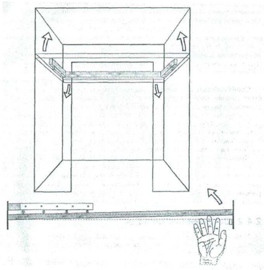
Мал. 26. Обладнання фальш панелі стелі у шафі
