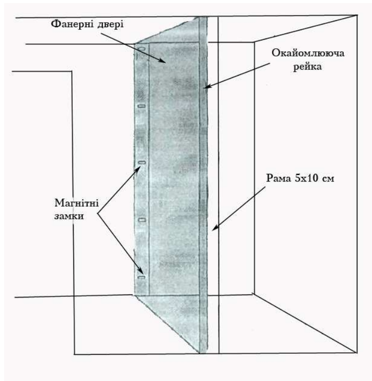
Мал. 25. Тайник у шафі
