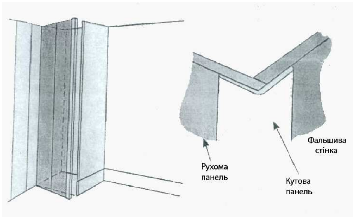
Мал. 27. Фальшивий кут
