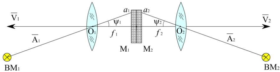
Рис. 3 Схема двоканального оптико-електронного приладу
