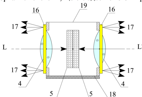
Рис. 2. Схема конструкції деформаційної марки
