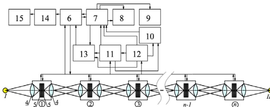
Рис. 1. Схема оптико-електронної створної лінії на лінійній ділянці інженерної споруди
