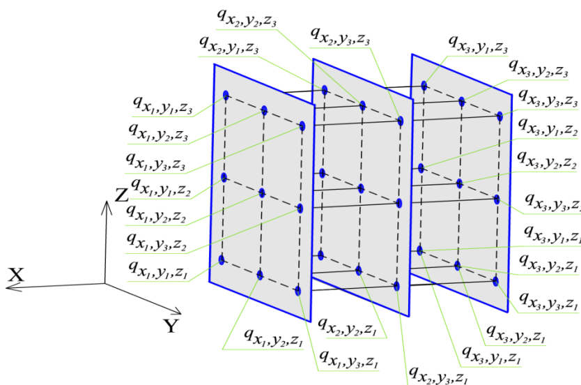
Рис. 5. Об’ємна просторова геодезична мережа ДМ
