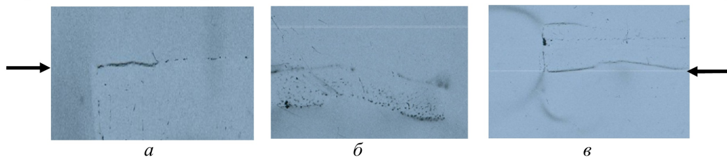
Рис. 1. Авторадіографічні відбитки зони з'єднання зразків у процесі зварювання алюмінію через фольгу: а – 2 шари; б – 4 шари; в – 6 шарів
