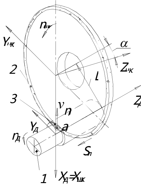
Рис. 4. Схема глибокого круглого шліфування зі схрещеними осями інструмента та деталі:
