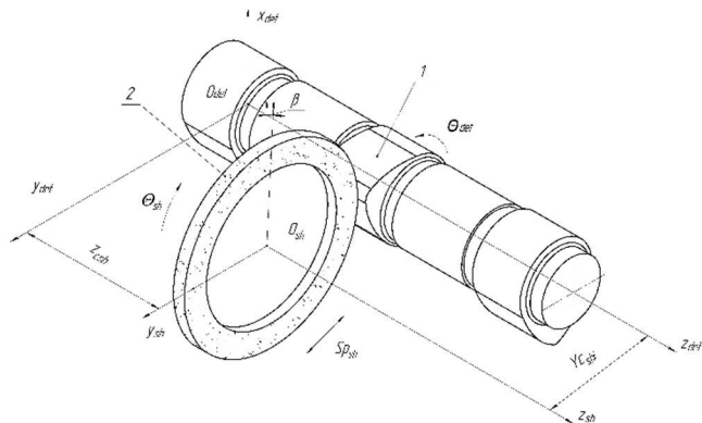
Рис. 1. Схема обробки розподільчого вала фірмою Junker
