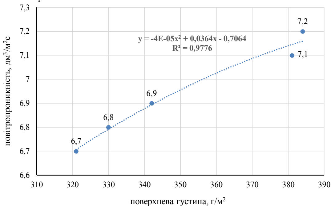
Рис. 3. Залежність повітропроникності дитячої куртки з пір'яно-пуховим наповнювачем (зразок 1) від поверхневої густини пакета
