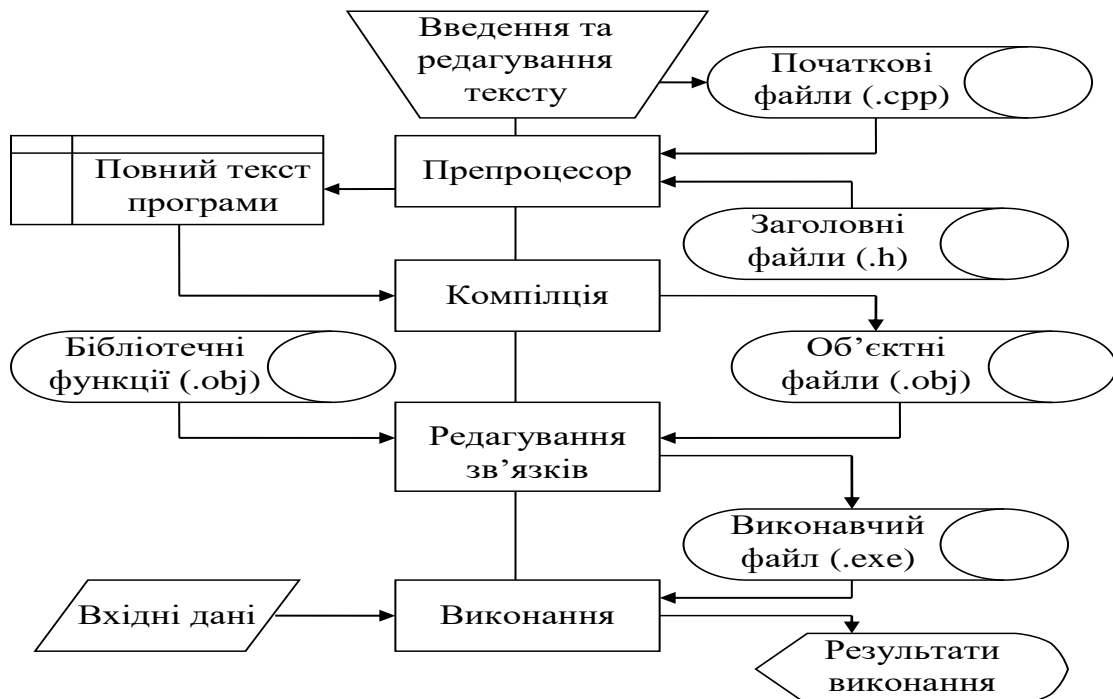
Рисунок 2.2 – Етапи виконання програми [1]
