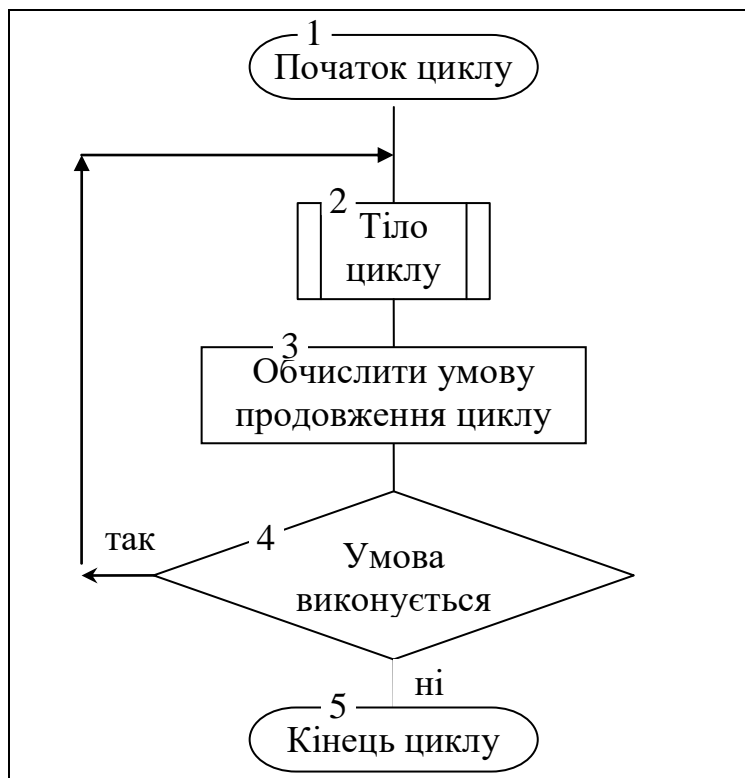
Рисунок 6.11 – Схема алгоритму виконання циклу do...while
