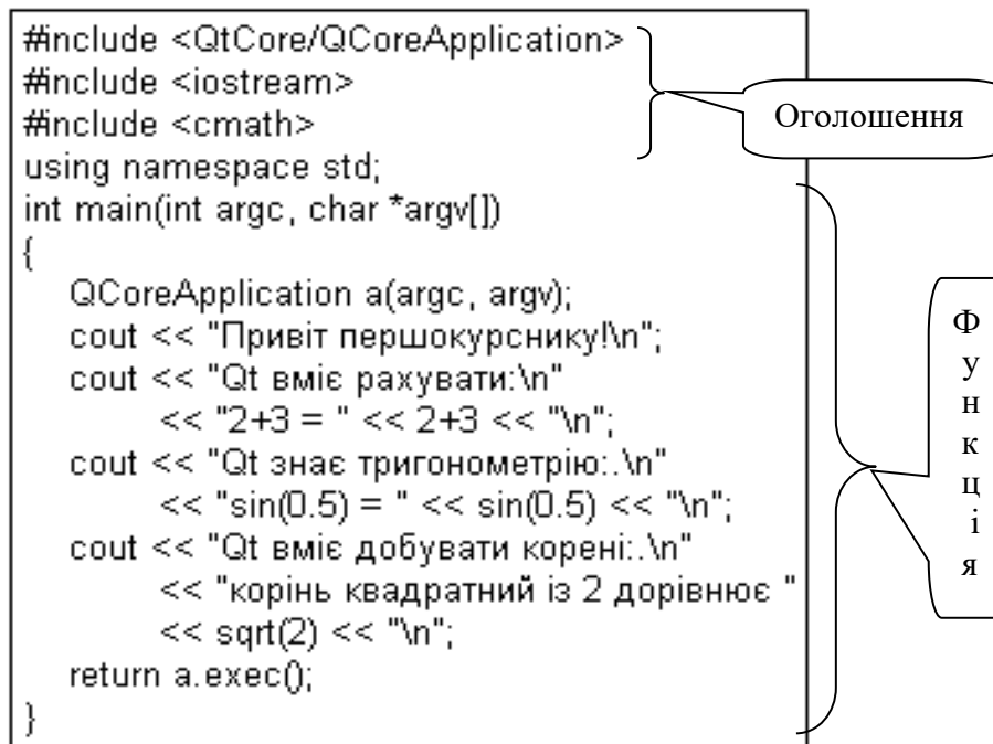
Рисунок 2.1 – Файл програми на С
