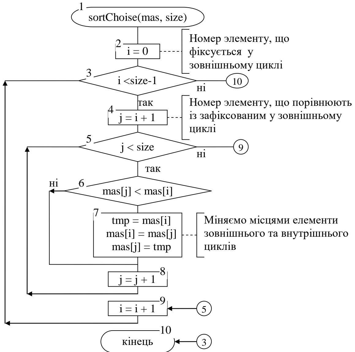
Рисунок 10.1 - Алгоритм сортування елементів масиву у зростаючому порядку за методом вибору
