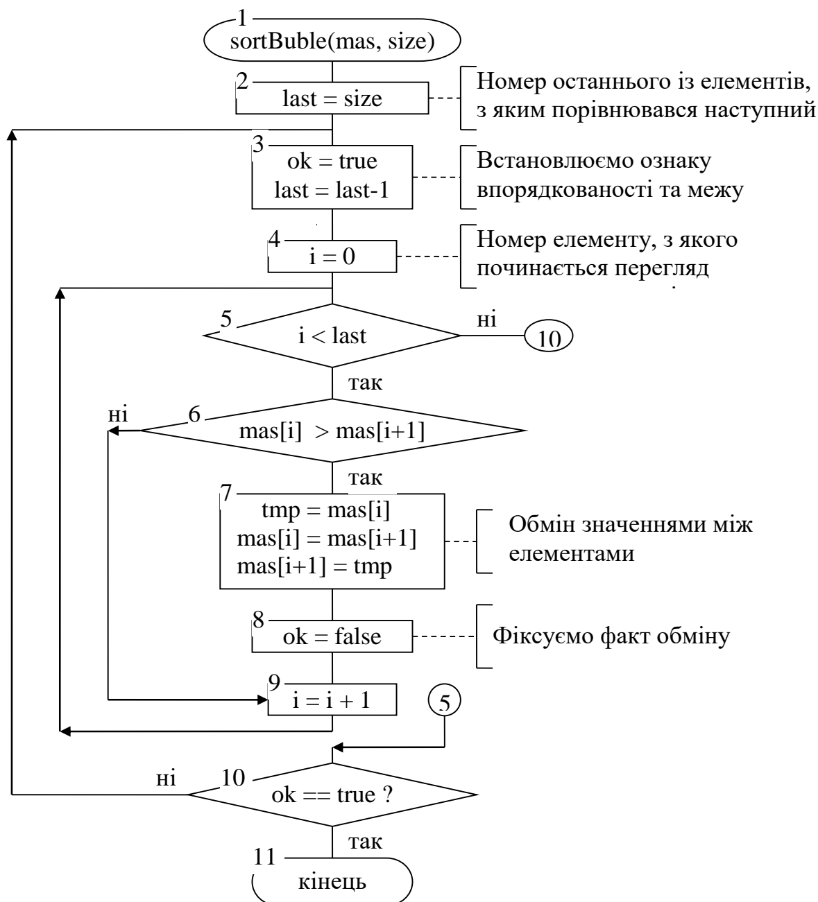
Рисунок 10.3 - Алгоритм сортування елементів масиву у зростаючому порядку за методом обміну
