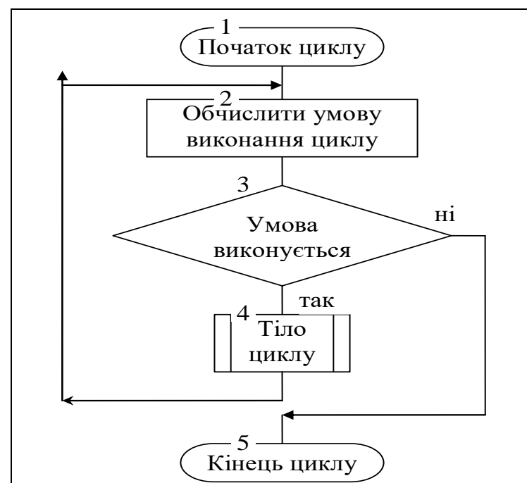
Рисунок 6.9 – Схема алгоритму виконання циклу while
