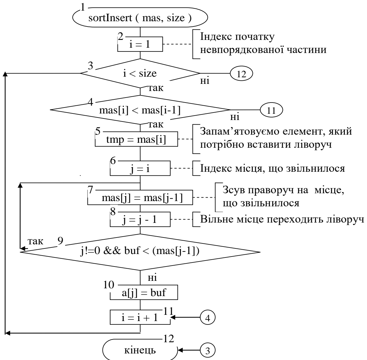
Рисунок 10.5 - Алгоритм сортування елементів масиву у зростаючому порядку за методом вставки
