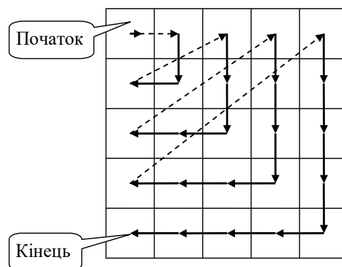
Рисунок 10.8 – Схема маршруту обходу матриці кутом униз і ліворуч, у напрямку головної діагоналі
