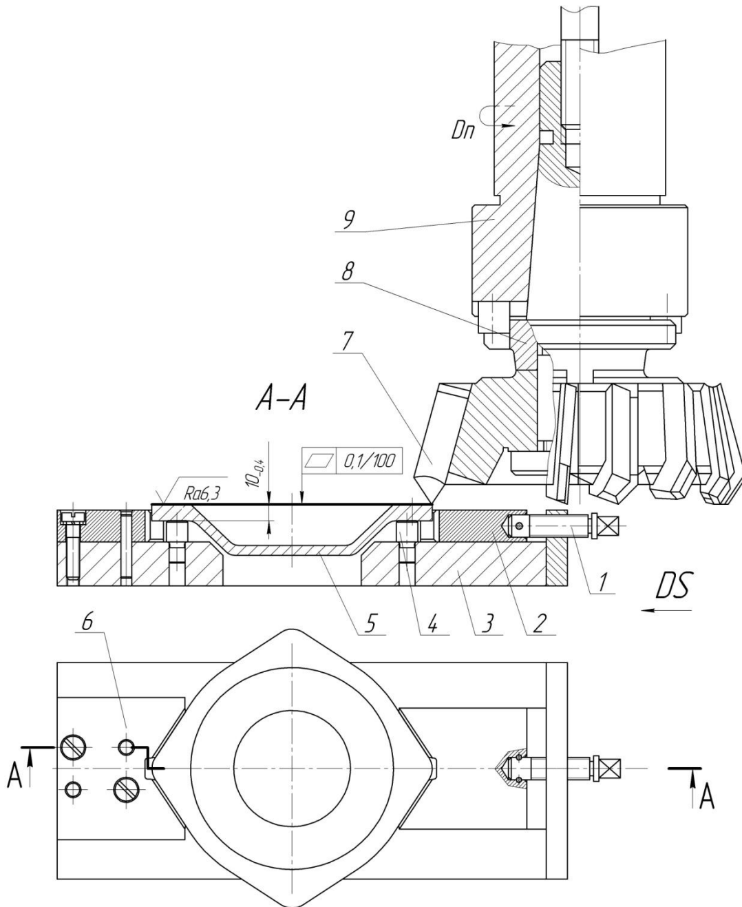
Рисунок 2.4 – Приклад схеми обробки площини кришки, витримуючи розмір 10_{-0,4} мм
