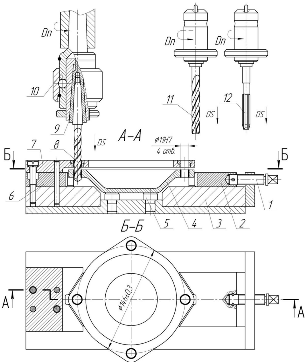
Рисунок 2.3 – Приклад схеми обробки отворів \text{Ø}11\text{H}7\text{мм}
