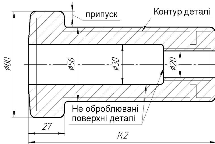
Рисунок 2.2 – Приклад виконання ескіза заготовки
