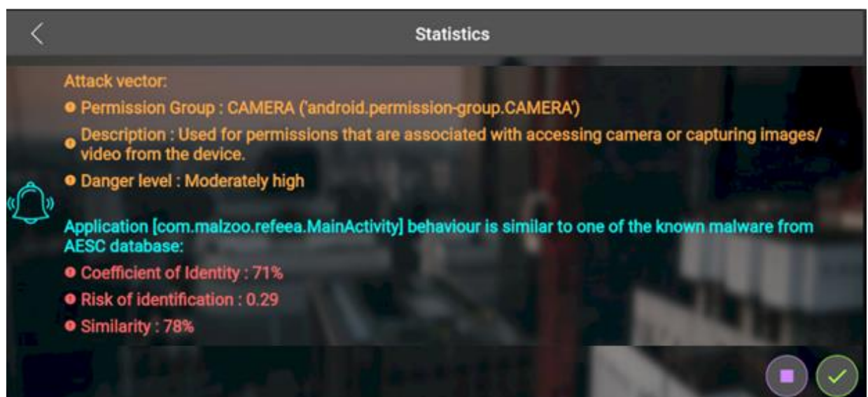
Рисунок 6 – Приклад нотифікації користувача
