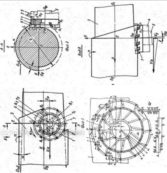
Спосіб фрезерування валів пат. 1042907, Петров В.И.
