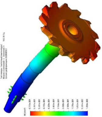
2-га власна частота і форма коливань
