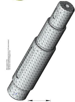
1-ша власна частота і форма коливань
