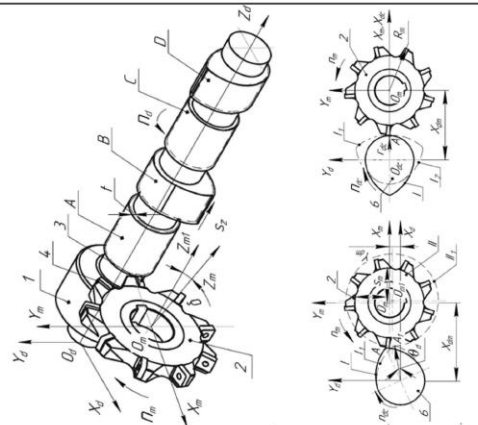
Схема фрезерування опорних шийок та кулачків розподільного вала за один установив Кальченко В.И., Кальченко В.В., Сіра Н.М.
