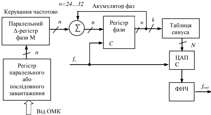
Рисунок 4 – Гнучка DDS-система
