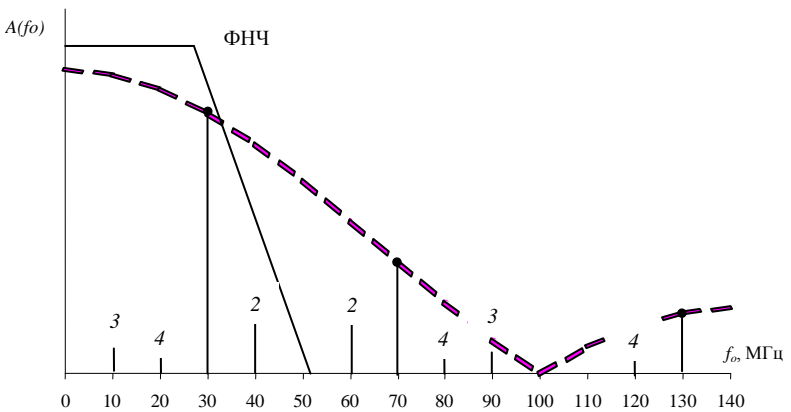
Рисунок 5 – Посадження спектрів в DDS-системі
