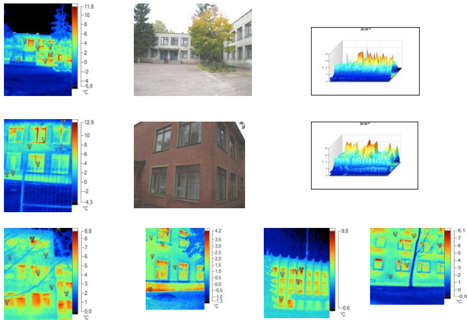
Рис. 6. Інфрачервоні термограми поверхні фасадів бюджетних будівель м. Чернігова
